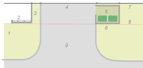
Vue en plan de l'organisation d'une entrée type
