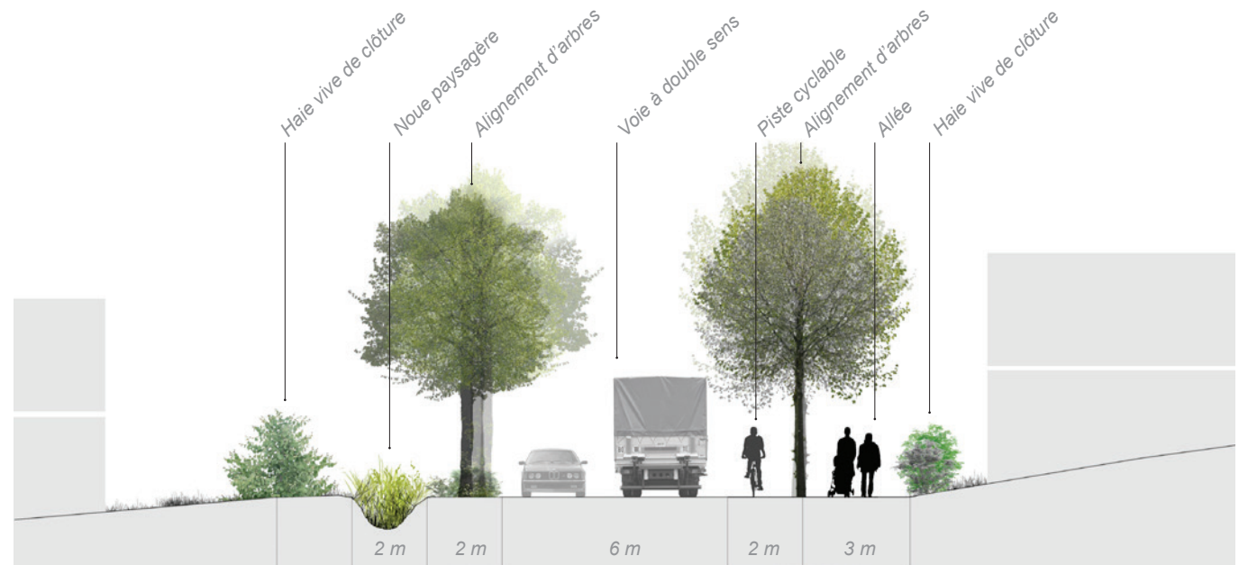
Profil type du nouvel axe
